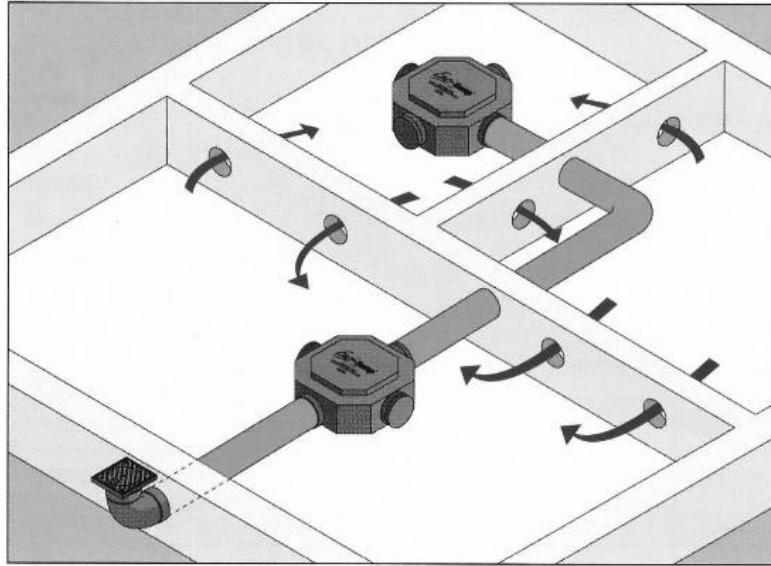
Фиг. 3.3. Сглобяеми радонови шахти
