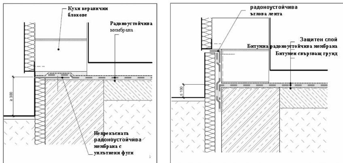
Фиг. 2.1. Прекъсване на въздушните прослойки между топлинната изолация по периметъра и основите на сграда
