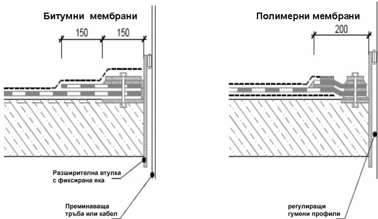
Фиг. 8.2. Въздухоплътност на отвори за сградни инсталации с дилатационно движение
